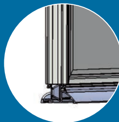
Etanchéité maximale : seuil en aluminium et panneau avec rejet d'eau avec son joint feutre
