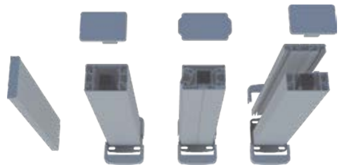
1/2 Poteau de départ 18,5 x 90 mm Poteau simple 90 x 60 mm Poteau orientable 90 x 55 mm Poteau multi-départ 90 x 60 mm
