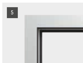
Dormant aluminium avec un double joint pour une meilleure étanchéité
