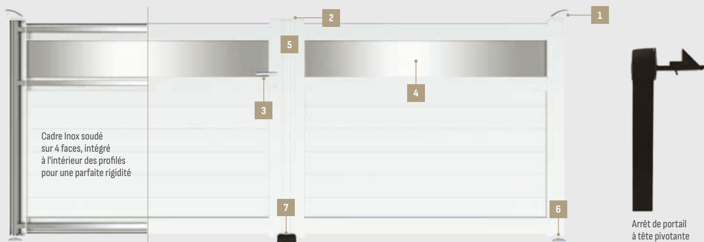
4 - Tôle standard en aluminium argenté épaisseur 2 mm
